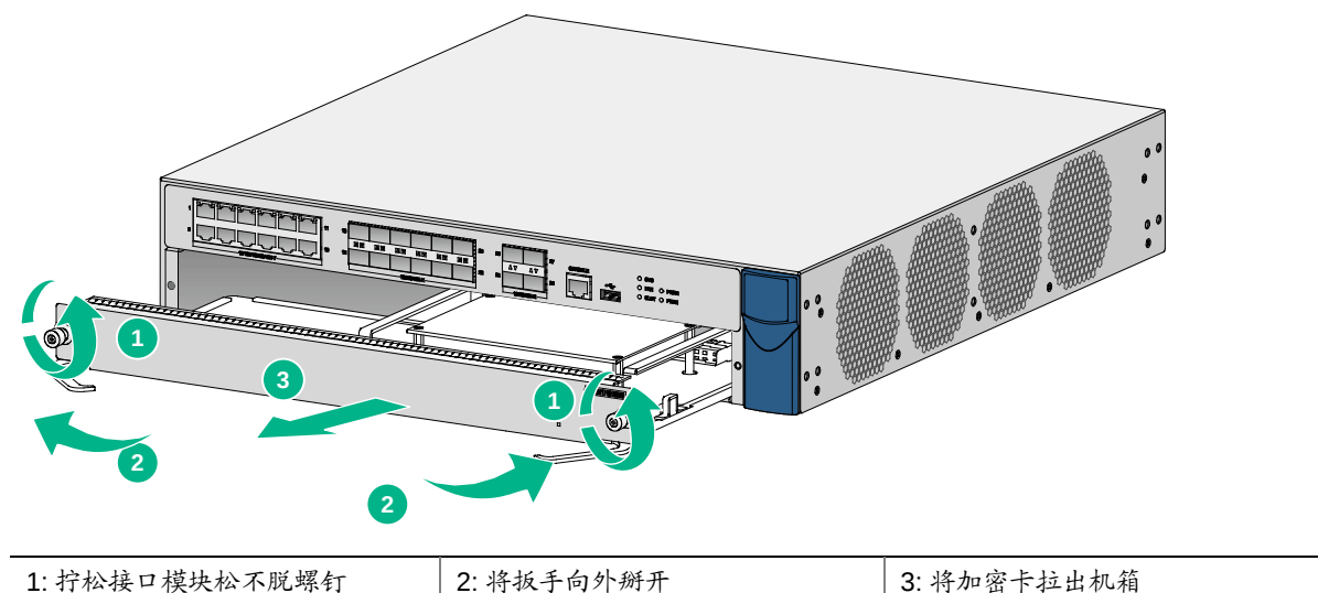
图4-2 拆卸 NSQM1F5KGMC 加密卡
