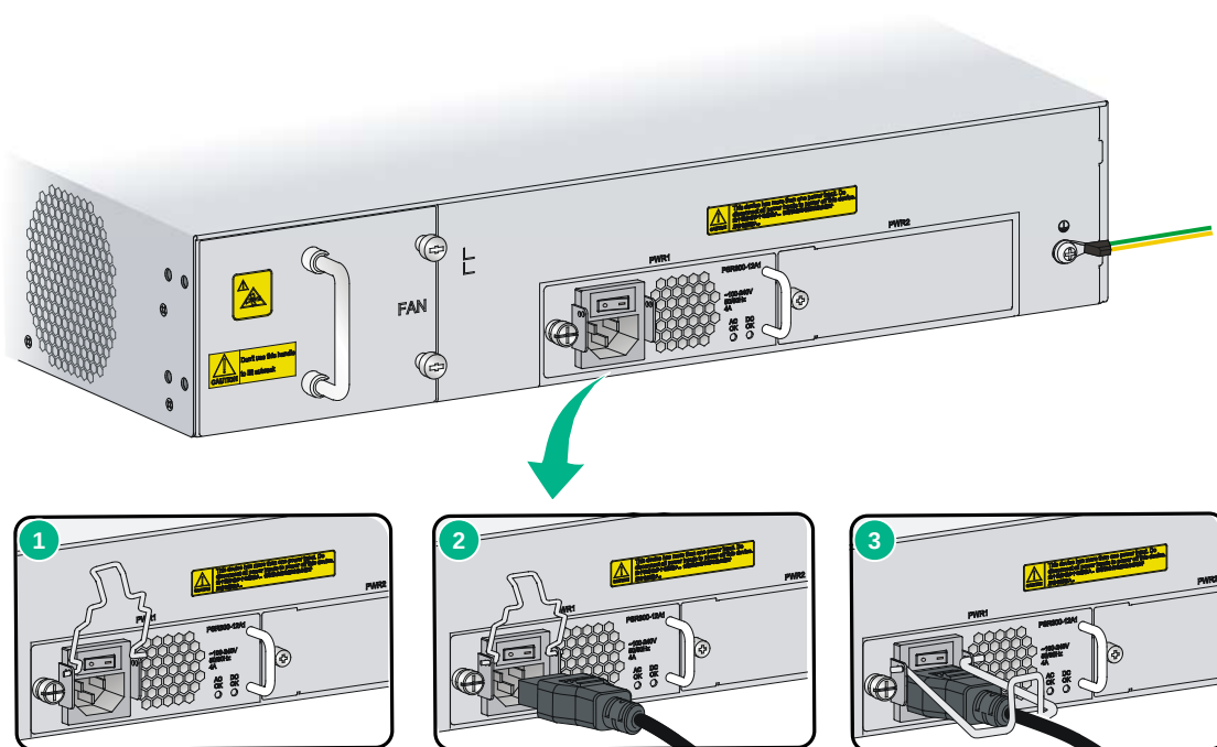
图2-14 连接交流电源线
