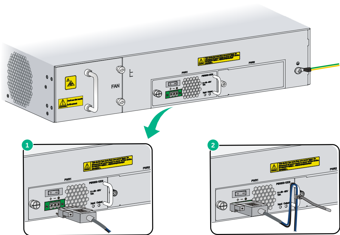
图2-15 连接直流电源线
