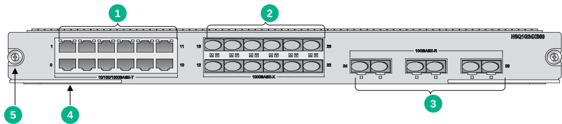
图A-3 NSQ1G24XS60 接口板正视图
