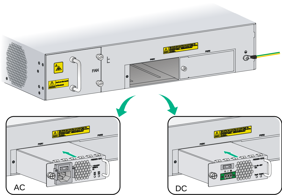
图2-9 安装电源模块
