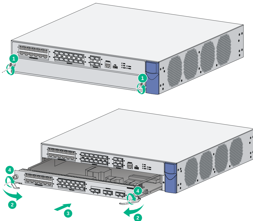
图2-10 安装 NSQ1G24XS60 接口模块
