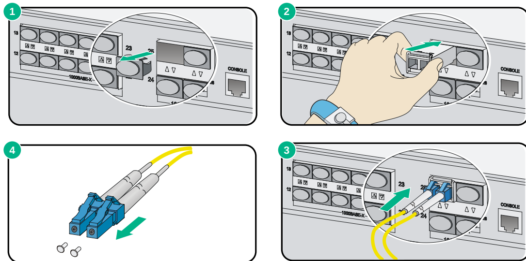
图2-13 连接光纤
